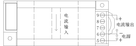
图 5、CE-IJ03-***BS2/ CE-IJ03-***ES3 电流输出接线参考
