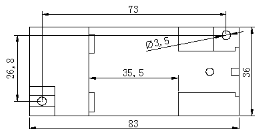
图 9、安装尺寸图
