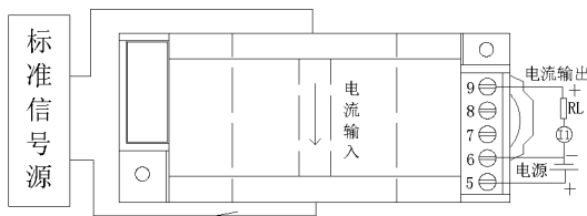
图 10 电流输出产品精度度试验接线图
